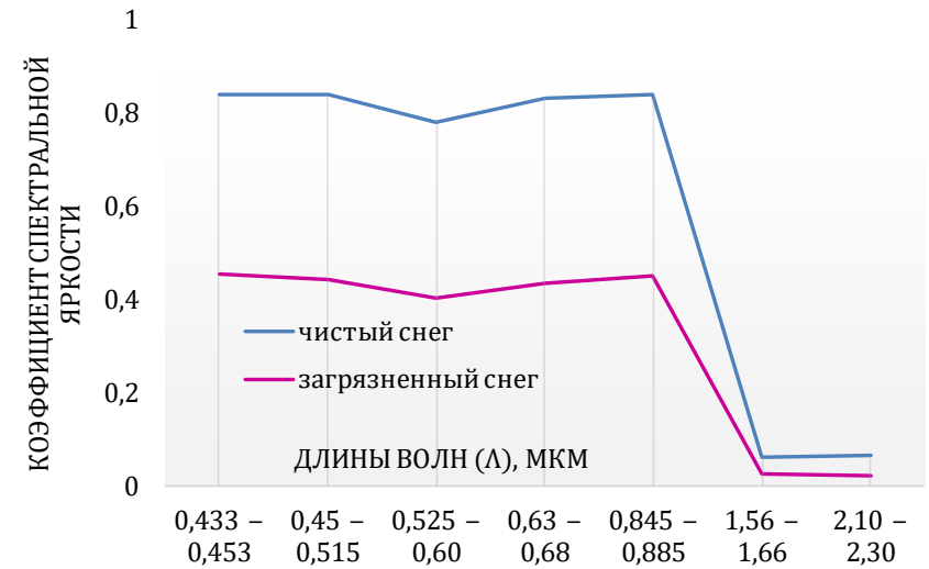
Рис. 3.3.5. Кривые спектральной отражательной способности чистого и загрязненного снежного покрова, построенные по снимку Landsat-8
